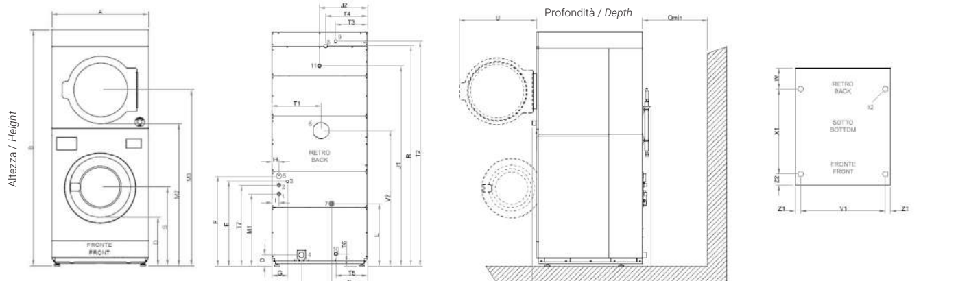
Pos. 1 - Acqua fredda lavatrice / Washing machine cold water Ø 3/4"; Pos. 2 - Acqua calda lavatrice / Washing machine hot water Ø 3/4"; Pos. 3 - Vapore diretto lavatrice (macchine vapore) / Washing machine direct steam (only steam heated machine); Pos. 4 - Scarico acqua lavatrice / Washing machine water drain Ø 50 mm; Pos. 5 - Sfiato lavatrice / Washing machine Ø 50 mm; Pos. 6 - Scarico aria umida e fumi (essiccatoio) / Humid air and smoke exit (Dryer) TDM 1111 Ø 100 mm, TDM 1818 Ø 150 mm; Pos. 7 - Alimentazione elettrica (presa unica) / Electrical power supply; Pos. 8 - Scarico condensa vapore essiccatoio (macchine vapore) / Dryer input steam (only steam heated machine) Ø 3/4" - 1"; Pos. 9 - Ingresso vapore essiccatoio (macchine vapore) / Dryer input steam (only steam heated machine) Ø 3/4" - 1"; Pos. 10 - Scarico condensa lavatrice (macchine vapore diretto) / Washing machine steam drain (only direct steam heated machine); Pos. 11 - Connessione GAS (solo essiccatoi a GAS) / GAS supply (only GAS heated dryers) Ø 3/4"; Pos. 12 - 4 Piedini macchina "M10" / 4 "M10" feet - 100 mm = 3.93 inch. - fattore di conversione 1 / 25,4 \ factor conversion 1 / 25,4
