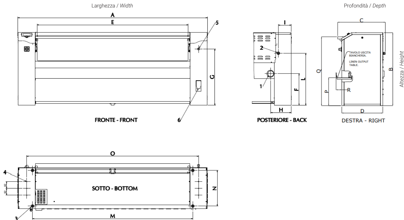
Pos. 1 - Scarico aria umida \ Humid air; Pos. 2 - Alimentazione elettrica / Electrical power supply; Pos. 3 - 4 Piedini (M10) / 4 Feet (M10); Pos. 4 - Fissaggio al suolo (Ø 13mm) / Fixing to the ground (Ø 13mm); Pos. 5 - Pulsante di emergenza / Emergency button; Pos. 6 - Sgancio di sicurezza conca / Chest safety release;
